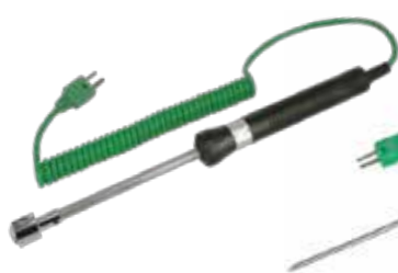
Termopar de contato tipo K | ITTPKCONT
